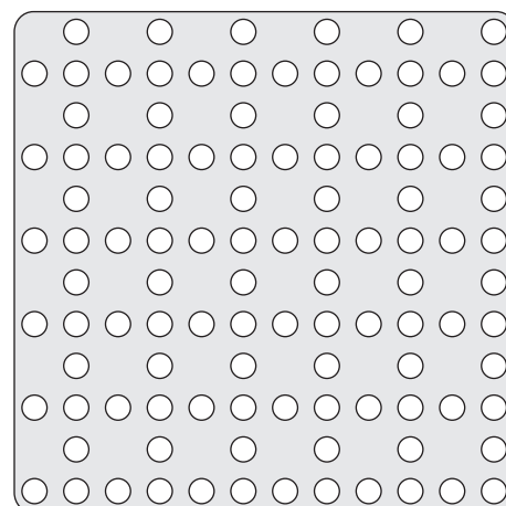
A6 Děrování pr.3mm, t = 5mm, t = 10mm, řadové
