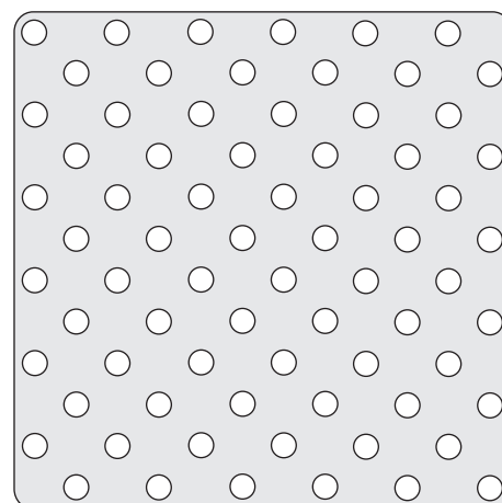
A4 Děrování pr.3mm, t = 10mm, přesazené
