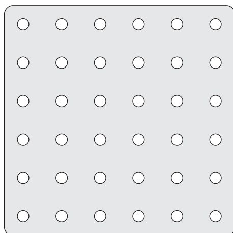
A3 Děrování pr.3mm, t = 10mm, řadové
