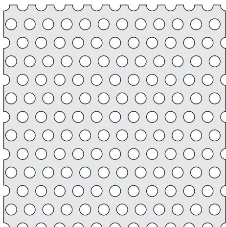
B1 Děrování pr.3mm, t = 5mm, přesazené
