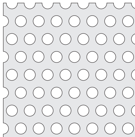
B2 Děrování pr.5mm, t = 8mm, přesazené
