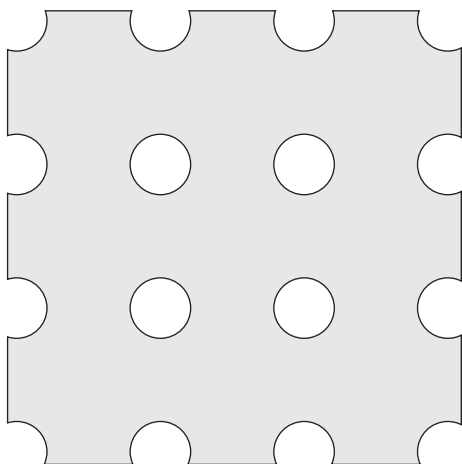
B3 Děrování pr.8mm, t = 19mm, řadové
