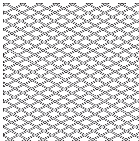
B4 Tahokov d = 6mm, š = 3mm, s = 0,5mm, m = 0,8mm
